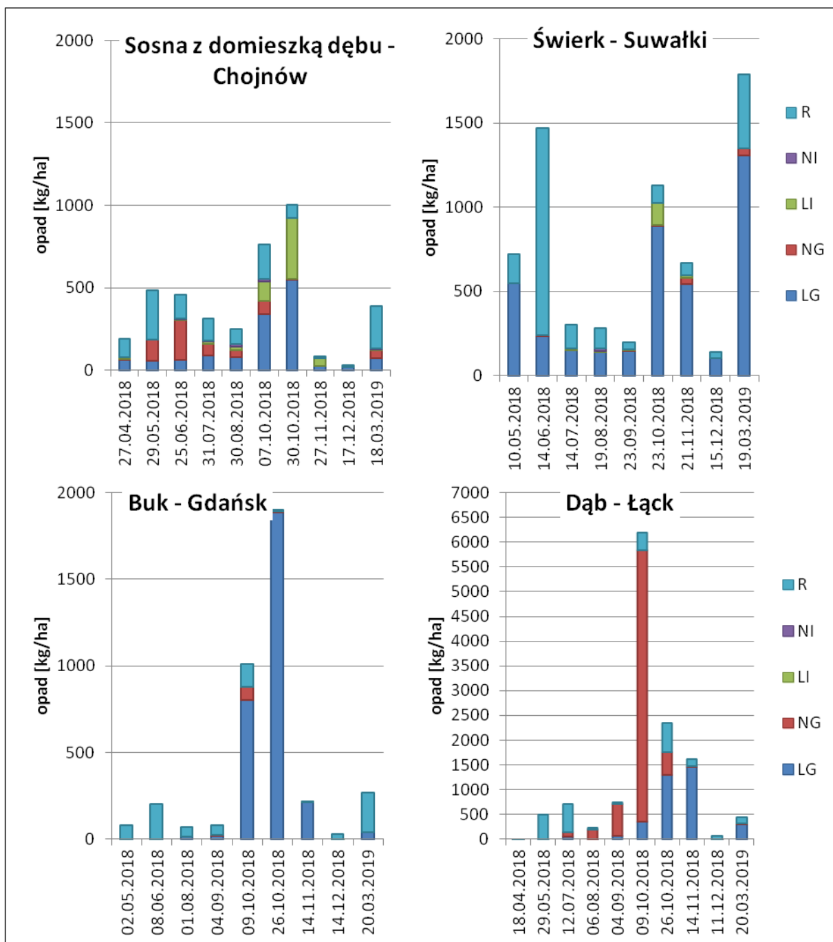
Rycina 141. Opad ścióły [ \text{kg ha}^{-1} ] w sezonie 2018/2019 w drzewostanach sosny (Nadl. Chojnów), świerka (Nadl. Suwałki), buka (Nadl. Gdańsk) i dębu (Nadl. Łąck). LG – liście gatunku głównego, NG – nasiona i owoce gatunku głównego, LI – liście innych gatunków, NI – nasiona innych gatunków, R – pozostałe resztki roślinne
