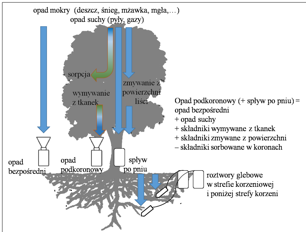
Rycina 126. Schemat koncepcyjny badań depozytu i przepływu składników w środowisku leśnym na SPO MI
